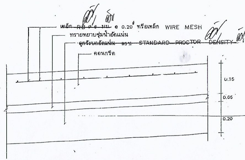
รายละเอียดของตะแกรงเหล็ก NOT TO SCALE
