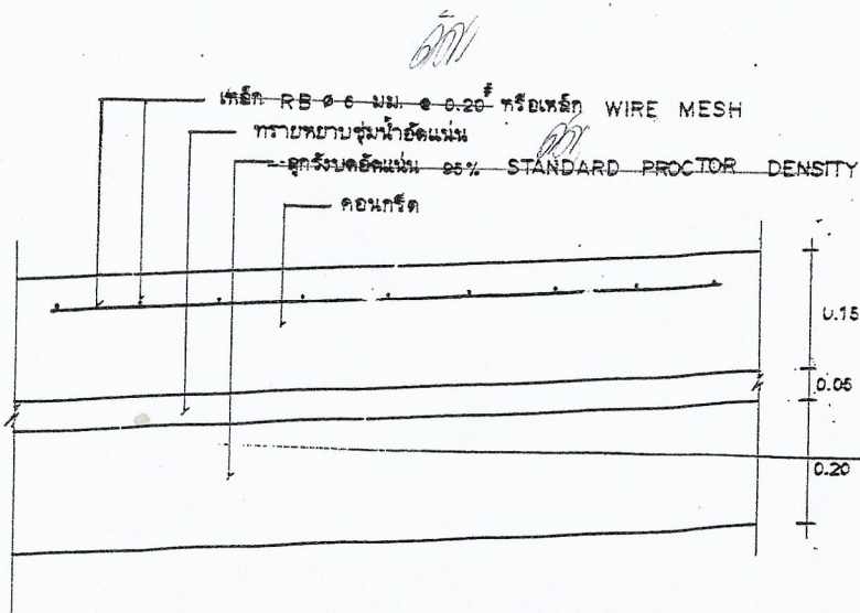
รายละเอียดคอนกรีตเสริมเหล็ก NOT TO SCALE
