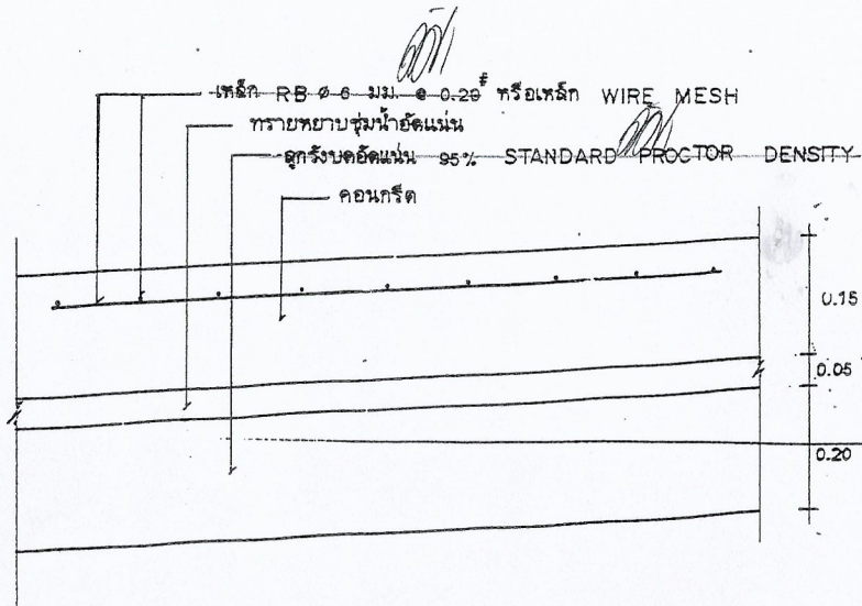
รายละเอียดค้ำคอนกรีตเสริมเหล็ก NOT TO SCALE
