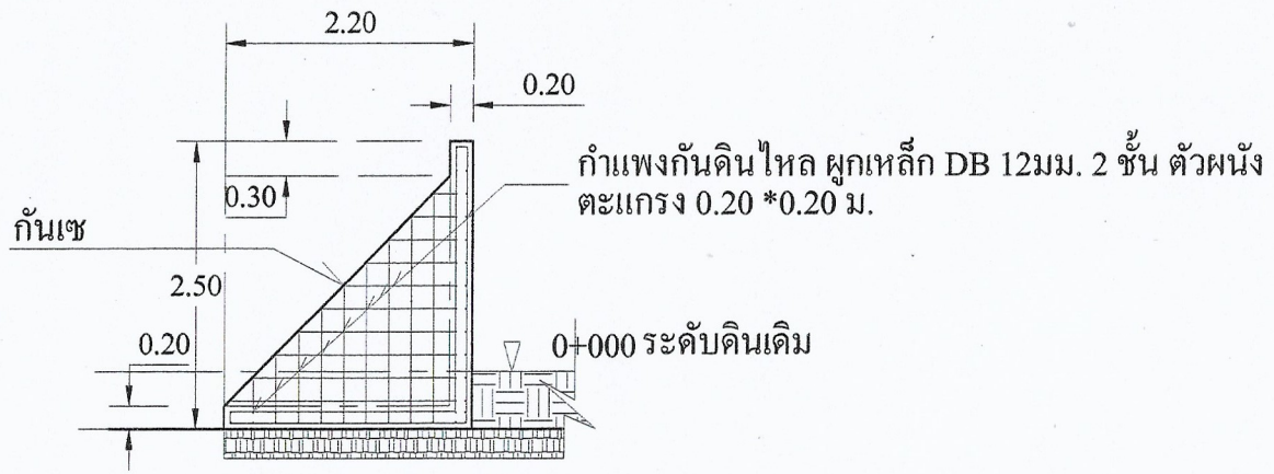
รูปตัด NO SCALE
