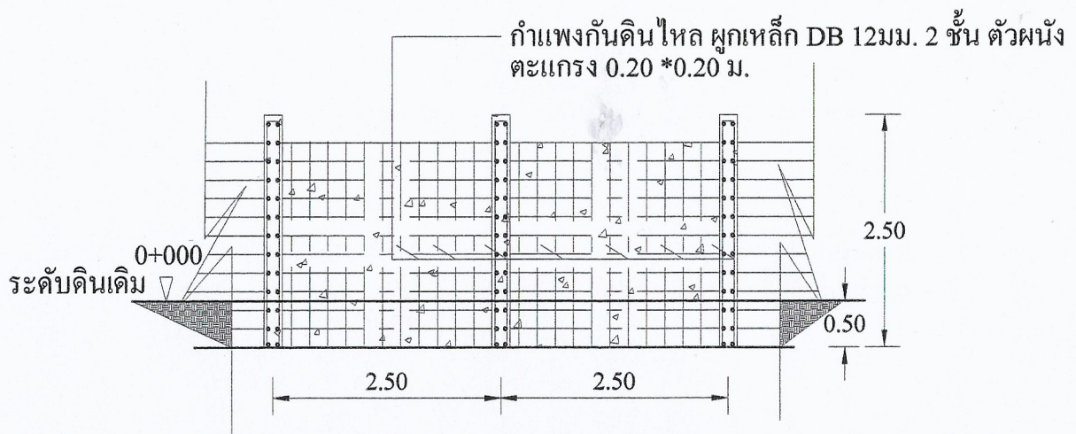
รูปตัด NO SCALE
