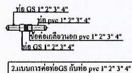
2.แบบการต่อท่อGS กับท่อ pvc 1" 2" 3" 4"
