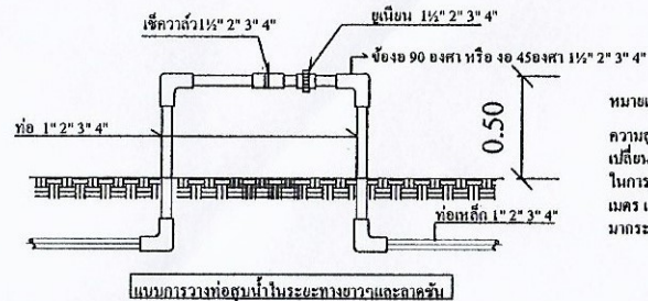
1.แบบการวางท่อสูบน้ำในระะทางยาวและลาดชัน
