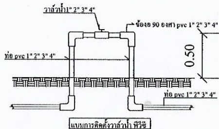
3.แบบการติดตั้งวาล์วน้ำ พีวีซี
