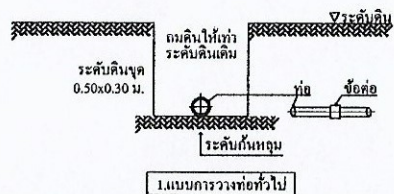
4.แบบการวางท่อทั่วไป
