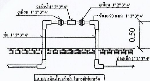
2.แบบการติดตั้งวาล์วน้ำ ในกรณีท่อเหล็ก
