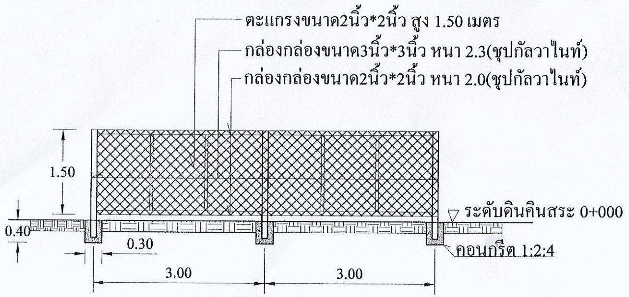
รูปตัดรั้วรอบคันสระ
