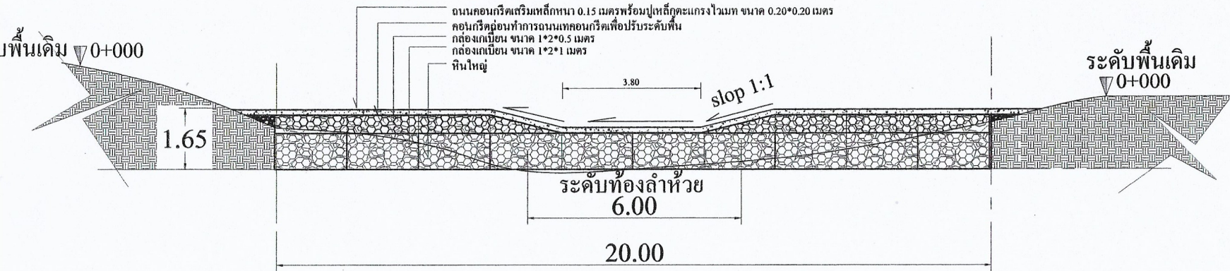
รูปตัด No SCALE
