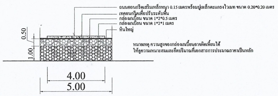
รูปตัด No SCALE
