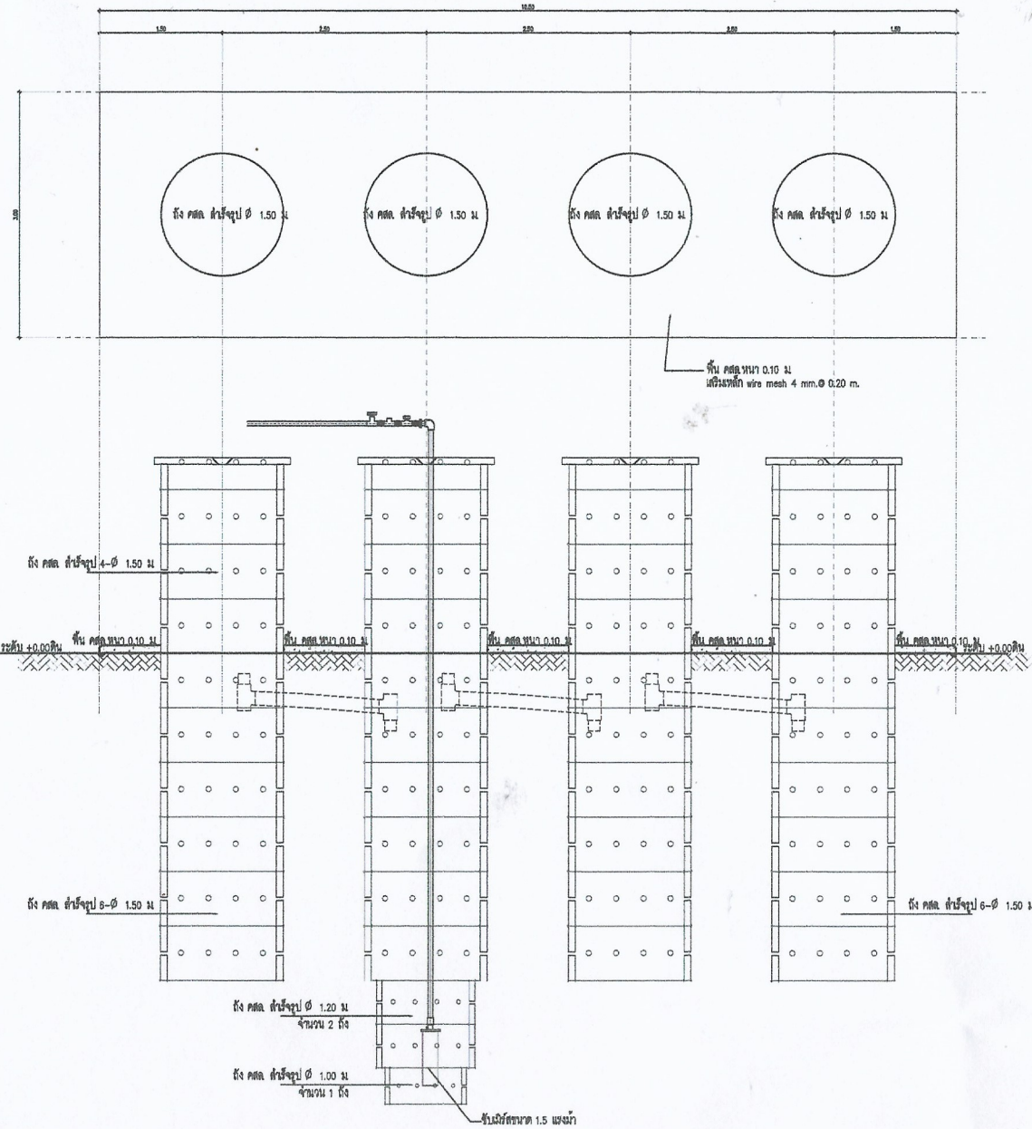
แบบขยาย บ่อรับน้ำ ขนาดท่อน 1: -
